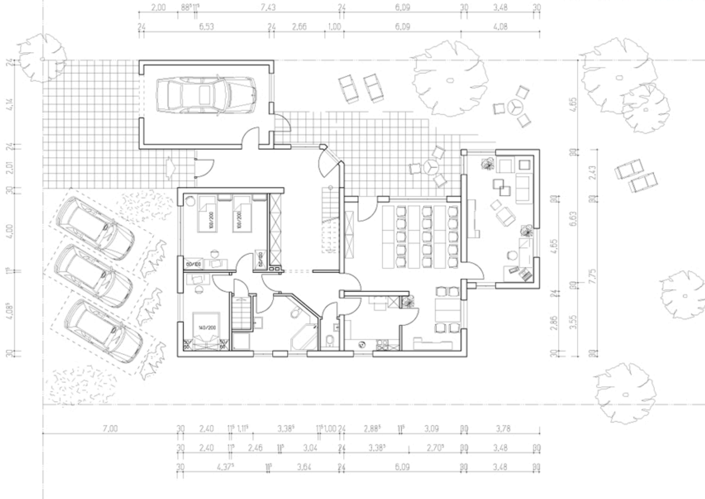
Grundriss Erdgeschoss Münsterbergerstrasse 13
